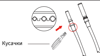
Рис. 3.4 Притисніть контактний штифт до дроту
